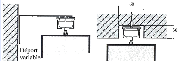
Pose de face avec équerres de déport renforcées
